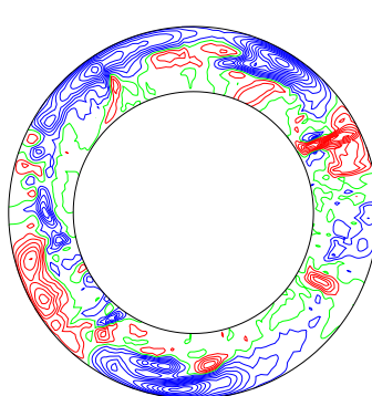
B_r (equat)
