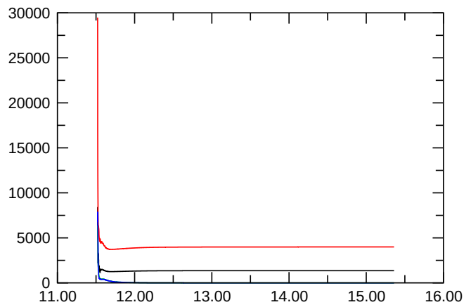
Nusselt Number
