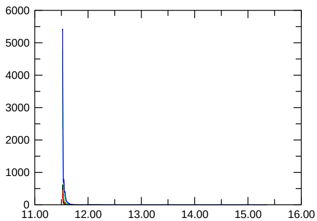
E_{\text{kin, asymm.}}
