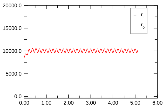
Nusselt Number
