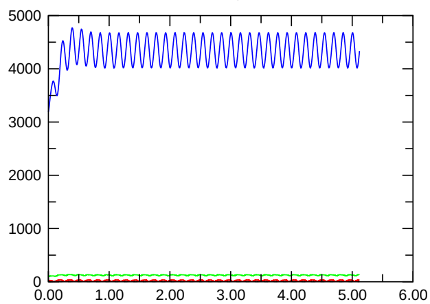
E_{\text{kin,asymm.}}
