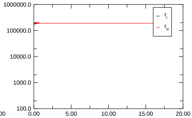
Nusselt Number
