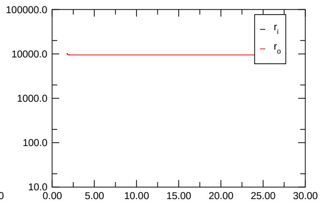
Nusselt Number
