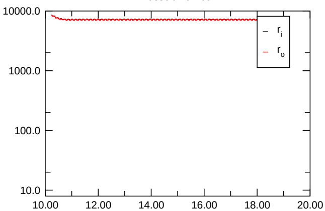
Nusselt Number
