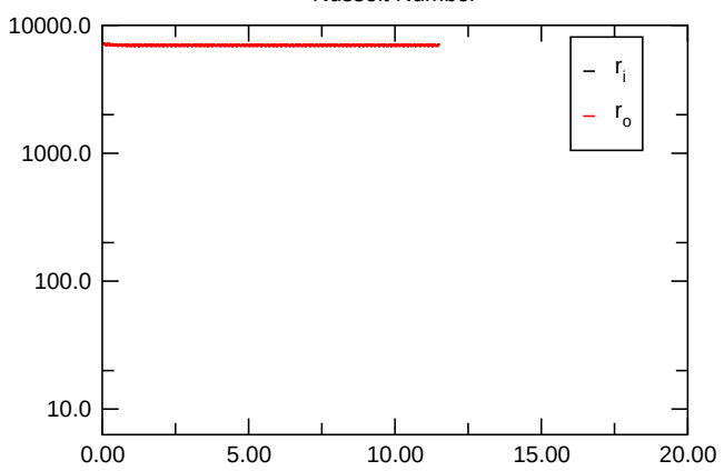
Nusselt Number
