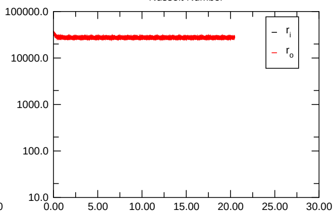
Nusselt Number
