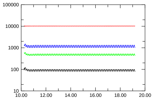
E_{\text{kin,symm.}}
