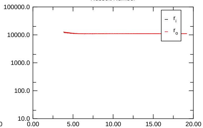
Nusselt Number
