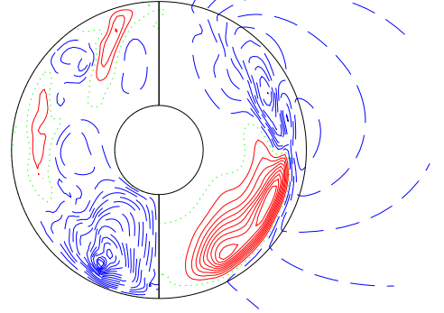
\bar{B}_\varphi & pol f-lines (mer)
