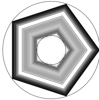
u_r (equat)
