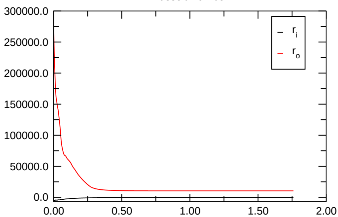
Nusselt Number
