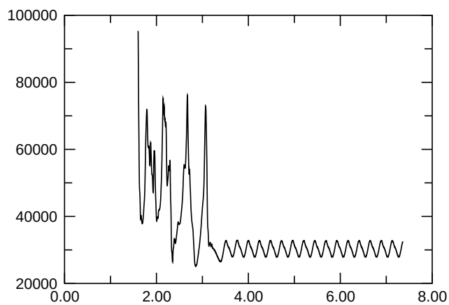
E_{\text{kin,asymm.}}
