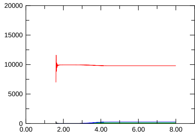
E_{\text{kin, symm.}}
