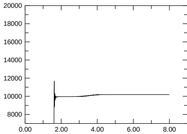
E_{\text{kin, asymm.}}
