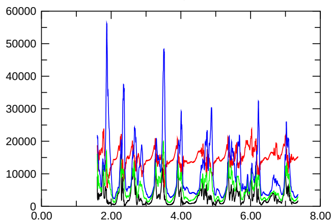
E_{\text{kin,symm.}}
