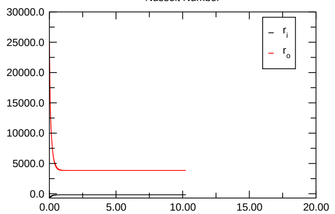
Nusselt Number
