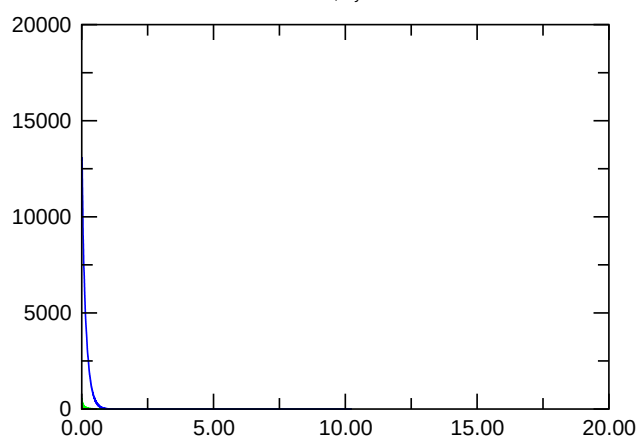
E_{\text{kin, asymm.}}
