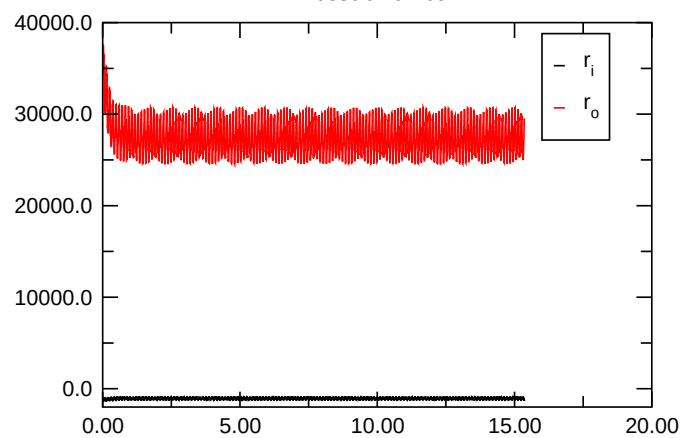
Nusselt Number
