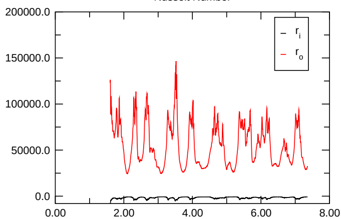
Nusselt Number
