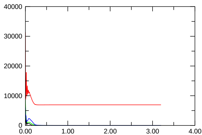
E_{\text{kin, symm.}}
