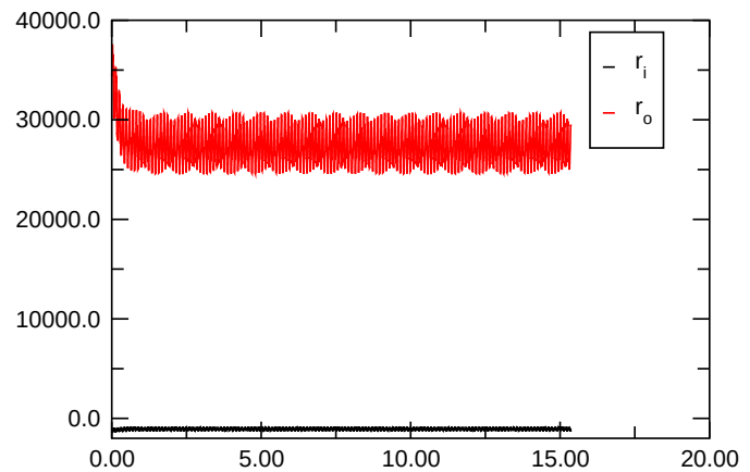
Nusselt Number
