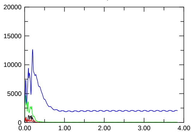
E_{\text{kin, asymm.}}
