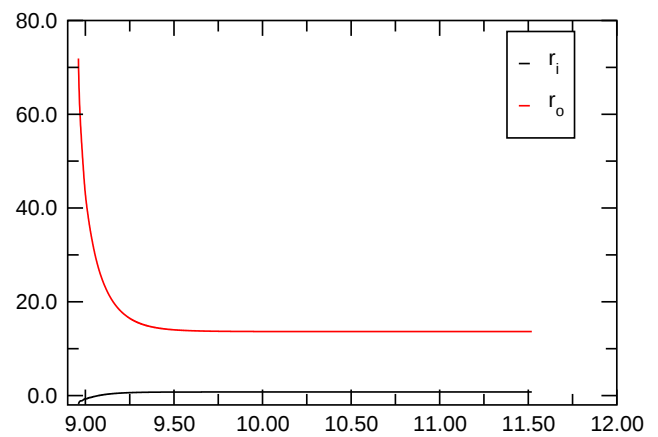
Nusselt Number
