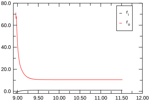
Nusselt Number
