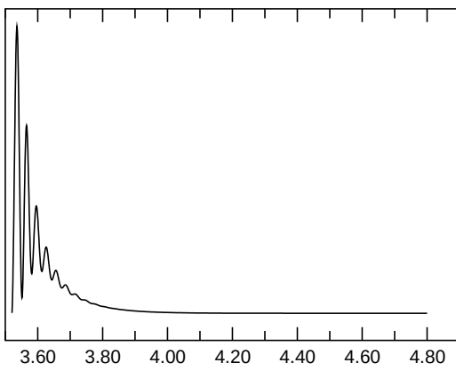
E_{\text{kin,asymm.}}
