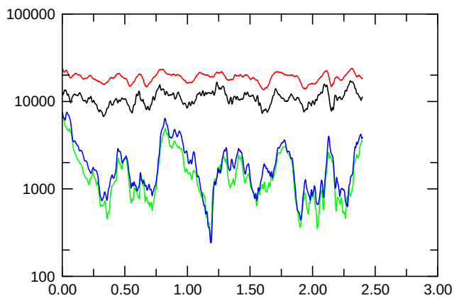
E_{\text{kin,symm.}}
