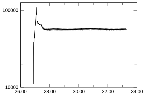
E_{\text{kin,asymm.}}
