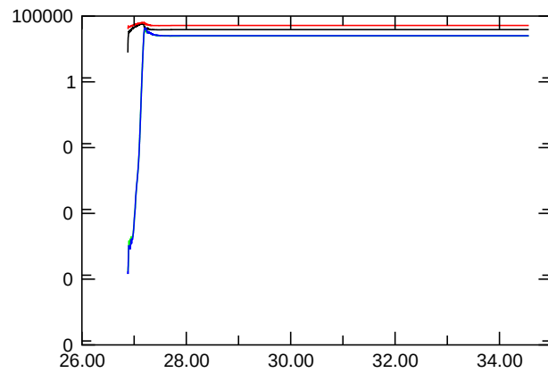
E_{\text{kin,symm.}}
