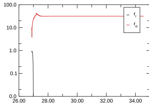
Nusselt Number
