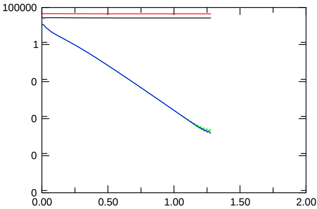
E_{\text{kin,symm.}}
