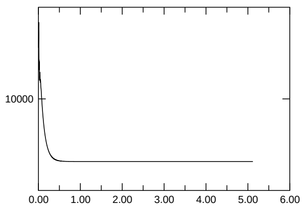
E_{\text{kin,asymm.}}
