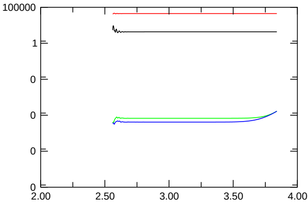
E_{\text{kin,symm.}}
