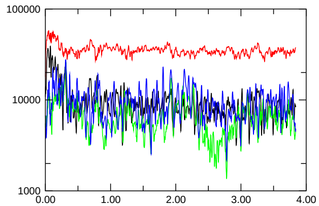
E_{\text{kin,symm.}}
