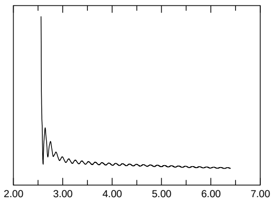
E_{\text{kin, asymm.}}
