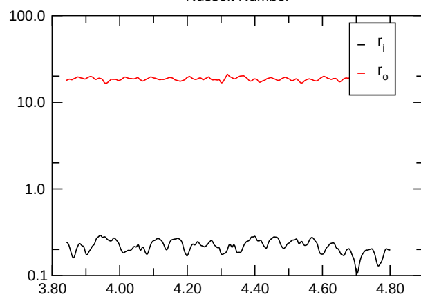
Nusselt Number
