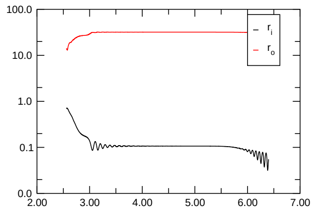
Nusselt Number
