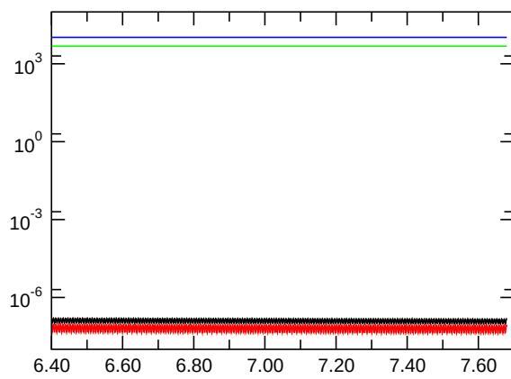
E_{\text{kin,asymm.}}
