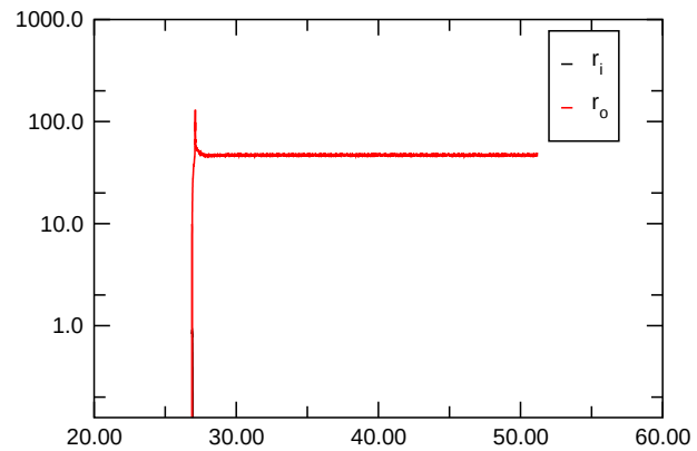
Nusselt Number
