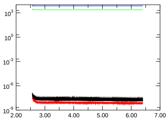
E_{\text{kin, asymm.}}
