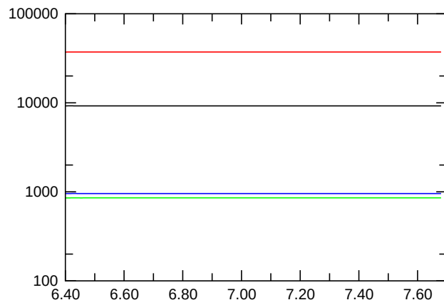
Nusselt Number
