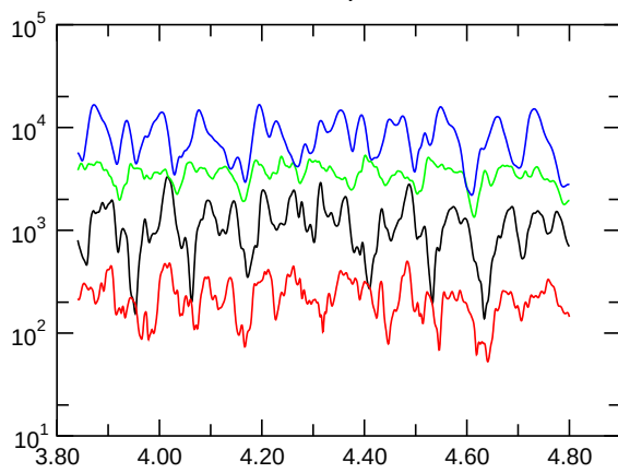
E_{\text{kin,asymm.}}
