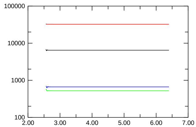
Nusselt Number
