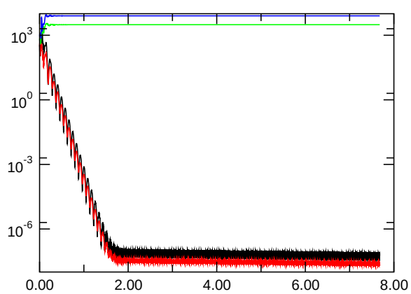
E_{\text{kin,asymm.}}
