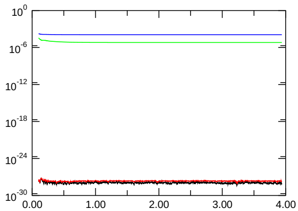
E_{\text{kin,asymm.}}
