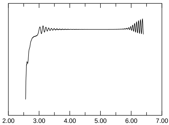
E_{\text{kin,asymm.}}
