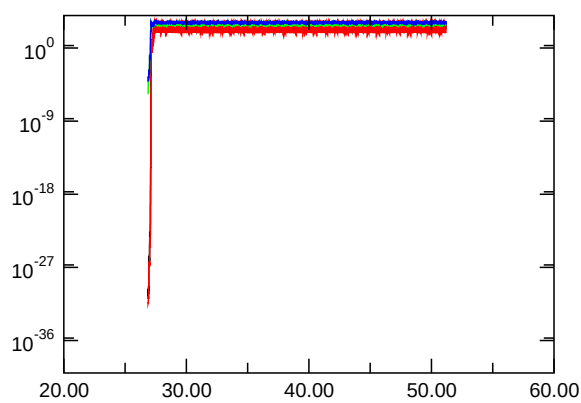
E_{\text{kin,asymm.}}
