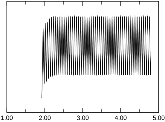
E_{\text{kin,asymm.}}
