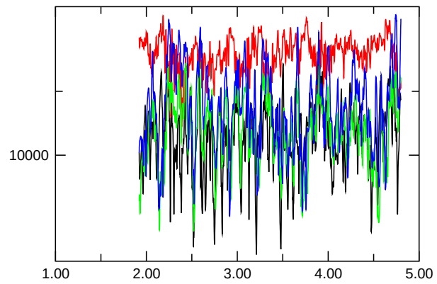
Nusselt Number
