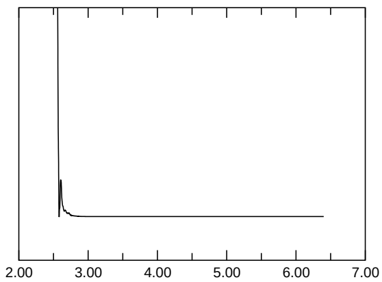
E_{\text{kin,asymm.}}
