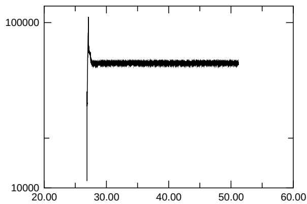
E_{\text{kin,asymm.}}
