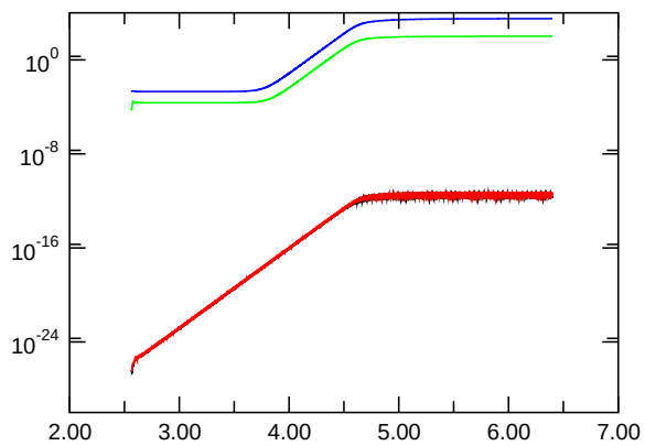
E_{\text{kin,asymm.}}
