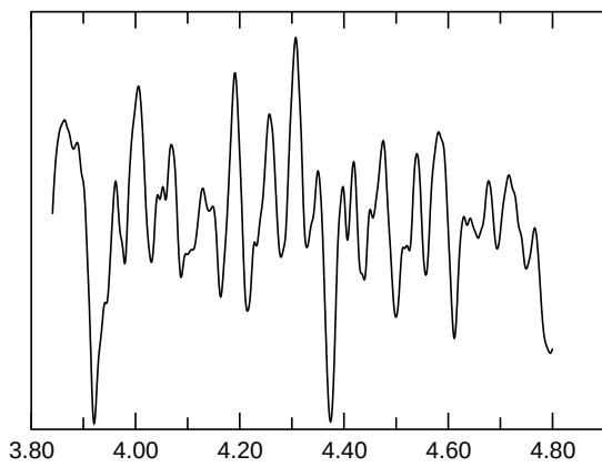
E_{\text{kin,asymm.}}
