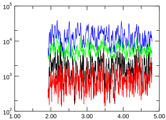
E_{\text{kin,asymm.}}
