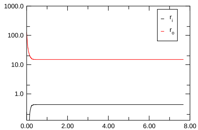
Nusselt Number
