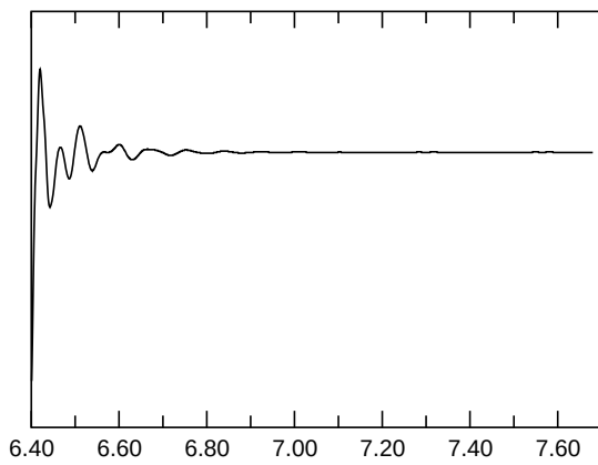
E_{\text{kin,asymm.}}
