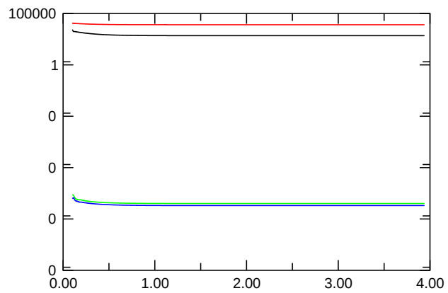
Nusselt Number
