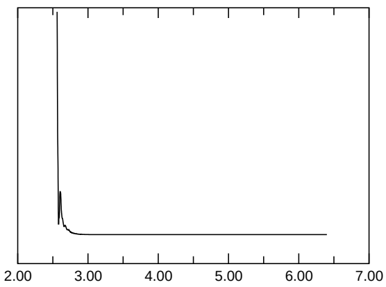
E_{\text{kin, asymm.}}
