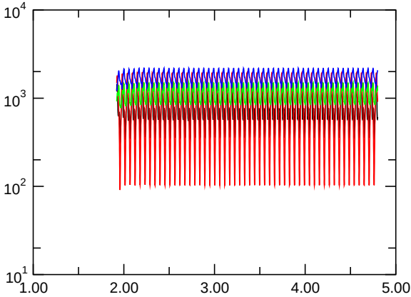
E_{\text{kin,asymm.}}
