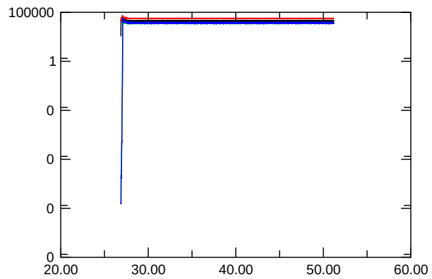
E_{\text{kin,symm.}}
