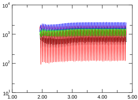
E_{\text{kin, asymm.}}
