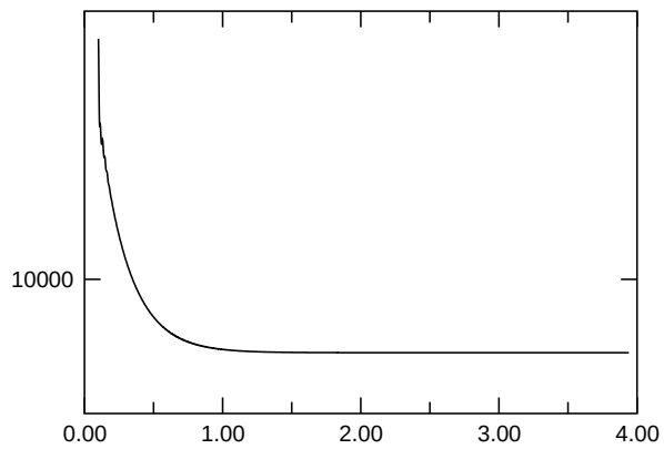
E_{\text{kin,asymm.}}
