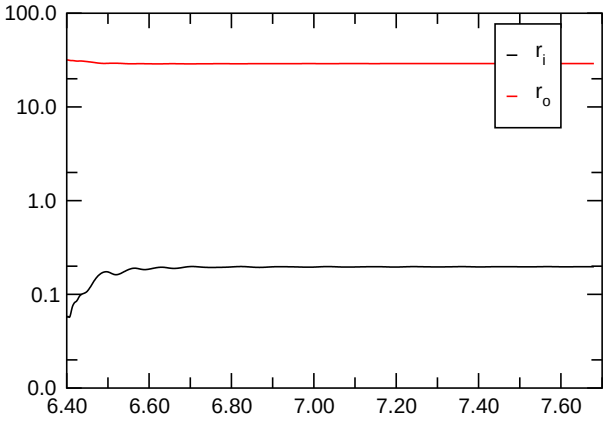
Nusselt Number
