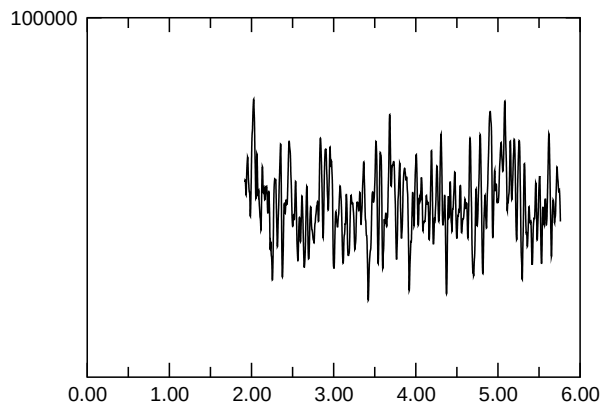
E_{\text{kin,asymm.}}
