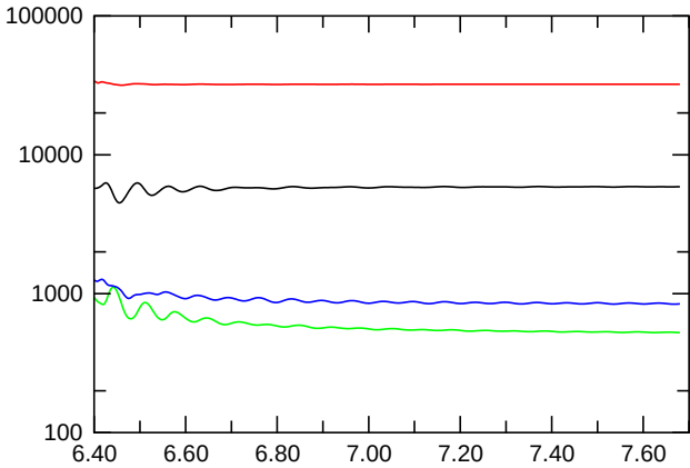
E_{\text{kin,symm.}}
