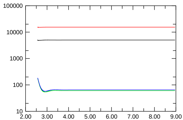
E_{\text{kin,symm.}}
