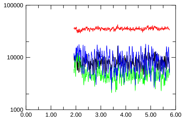
Nusselt Number
