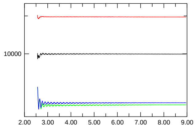
Nusselt Number
