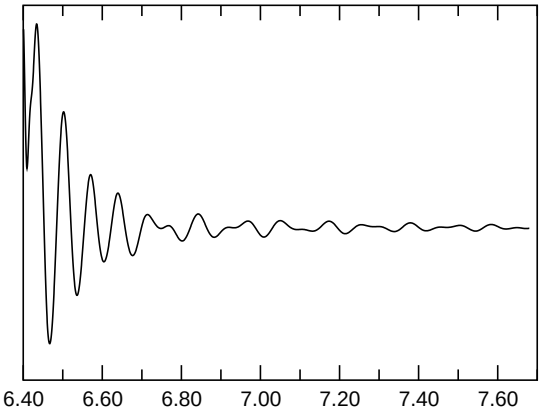
E_{\text{kin,asymm.}}
