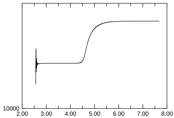
E_{\text{kin,asymm.}}
