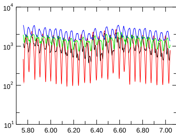
E_{\text{kin,asymm.}}
