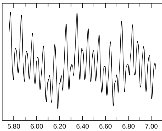
E_{\text{kin,asymm.}}
