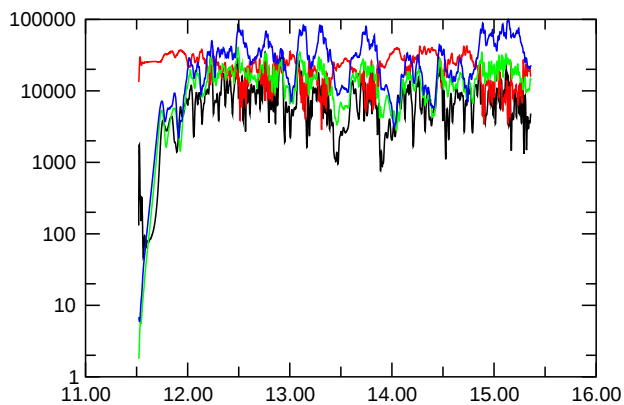
Nusselt Number
