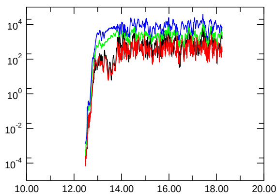
E_{\text{kin,asymm.}}
