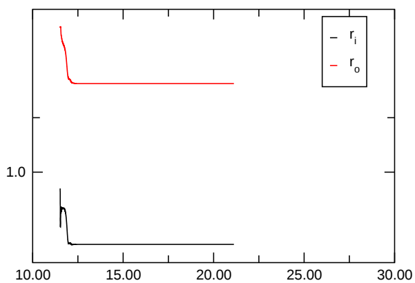
Nusselt Number
