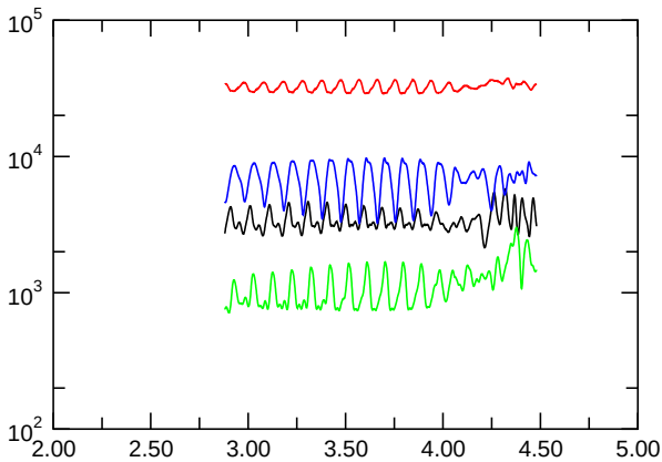
E_{kin,symm.}
