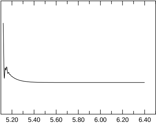
E_{\text{kin,asymm.}}
