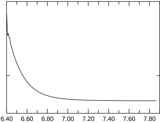
E_{\text{kin,asymm.}}
