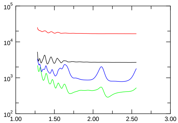
Nusselt Number
