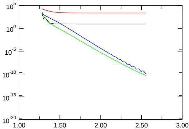
E_{\text{kin,symm.}}
