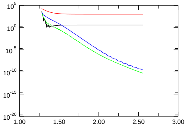
E_{kin,symm.}
