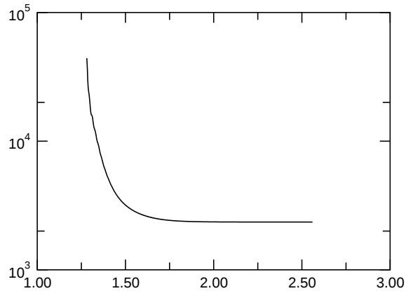
E_{\text{kin,asymm.}}
