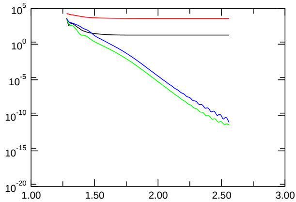
E_{\text{kin,symm.}}
