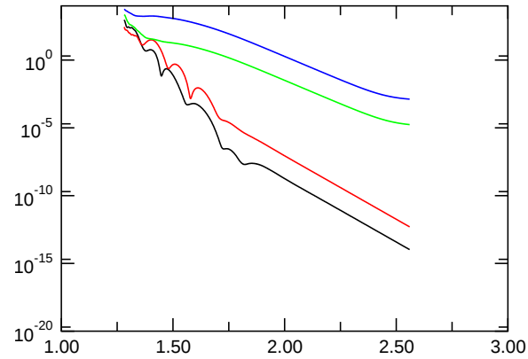
E_{\text{kin,asymm.}}
