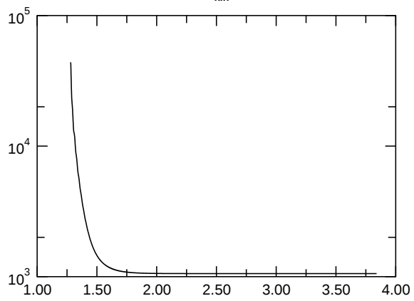
E_{\text{kin,asymm.}}
