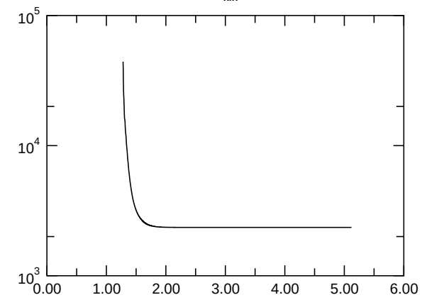
E_{\text{kin,asymm.}}
