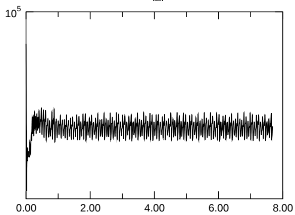
E_{\text{kin, asymm.}}
