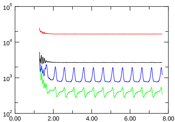
E_{\text{kin, symm.}}
