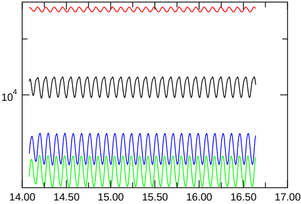
Nusselt Number
