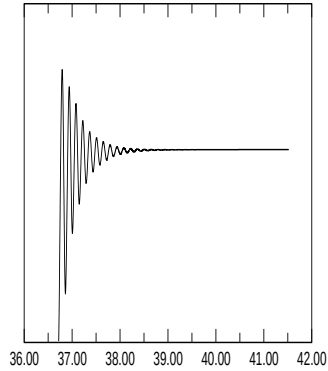
E_{\text{kin,asymm}}
