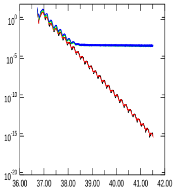
E_{\text{kin,asymm}}
