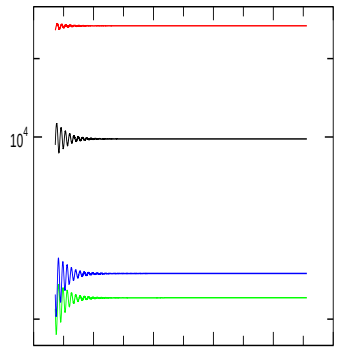
E_{\text{kin, symm.}}
