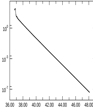
E_{magn,quadr.}
