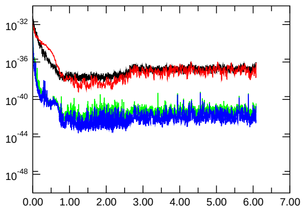
E_{\text{kin,asymm.}}
