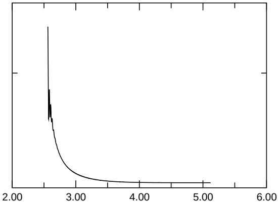
E_{\text{kin,asymm.}}
