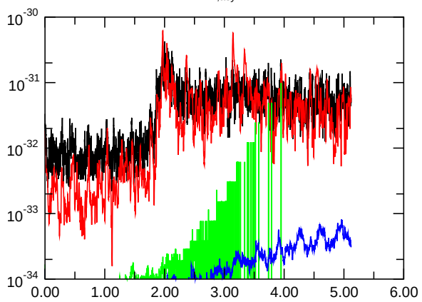
E_{\text{kin,asymm.}}
