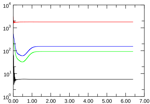
Nusselt Number
