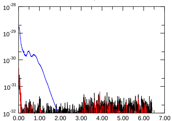
E_{\text{kin,asymm.}}
