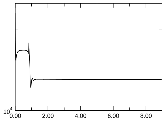
E_{\text{kin,asymm.}}
