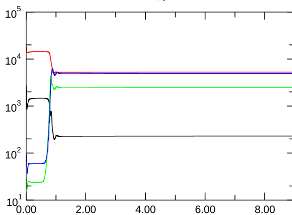
Nusselt Number
