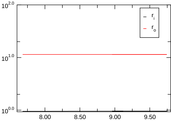
Nusselt Number
