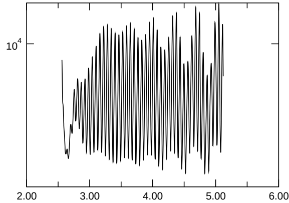
E_{\text{kin,asymm.}}
