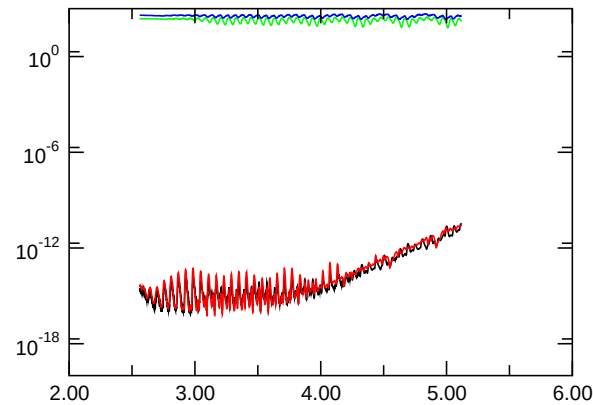
E_{\text{kin,asymm.}}
