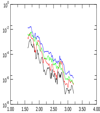
E_{\text{kin, asymm.}}
