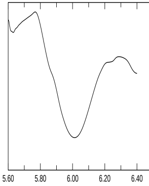
E_{magn, quadr.}
