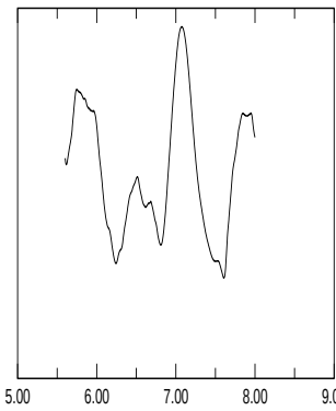
E_{magn,quadr.}
