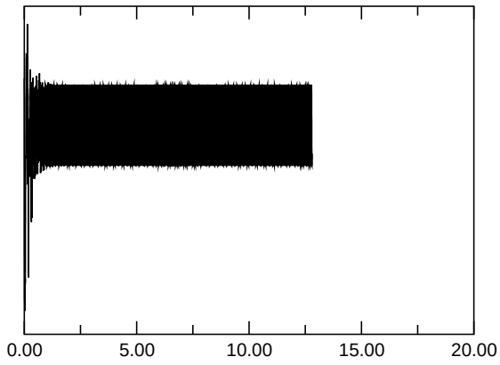
E_{\text{kin,asymm.}}
