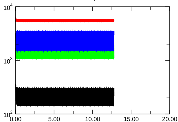
E_{\text{kin,symm.}}
