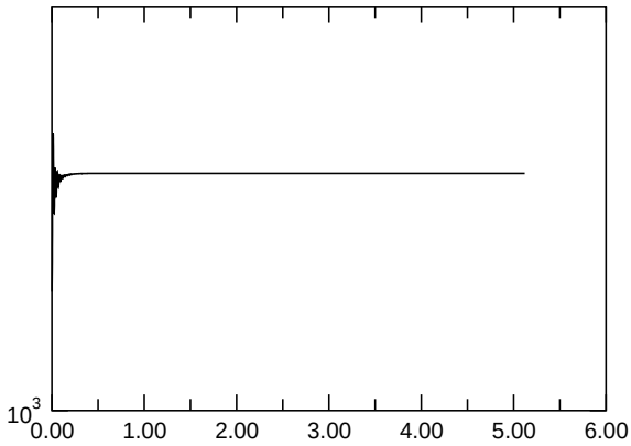
E_{\text{kin,asymm.}}
