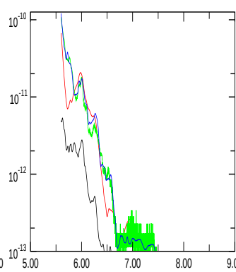
E_{magn,quadr.}
