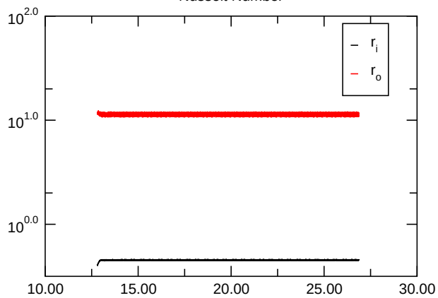
Nusselt Number
