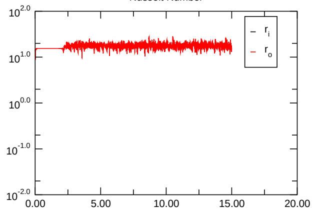
Nusselt Number
