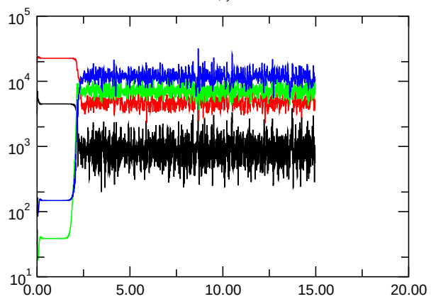
Nusselt Number
