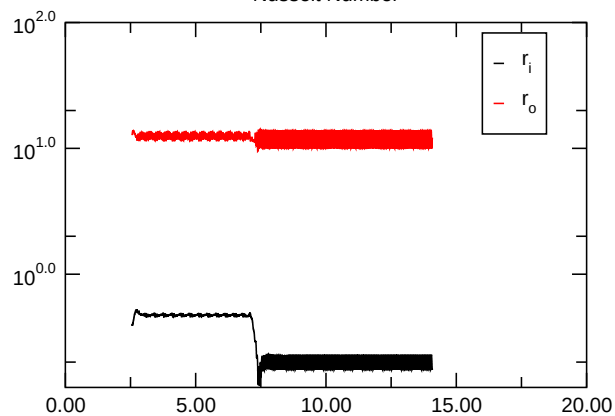
Nusselt Number
