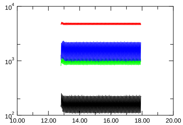
Nusselt Number
