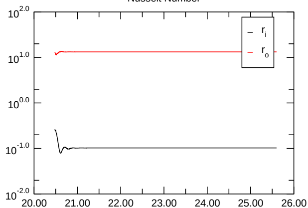
Nusselt Number
