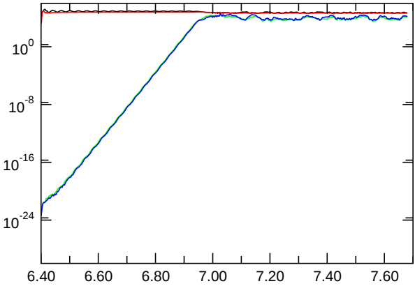
Nusselt Number
