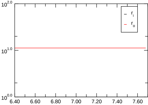
Nusselt Number
