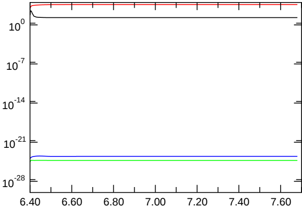
Nusselt Number
