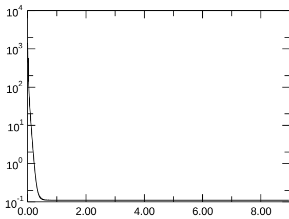
E_{\text{kin,asymm.}}
