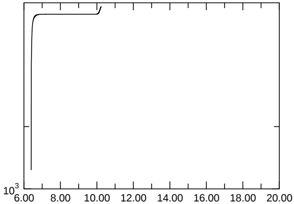
E_{\text{kin,asymm.}}
