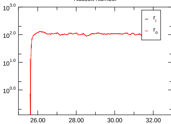
Nusselt Number
