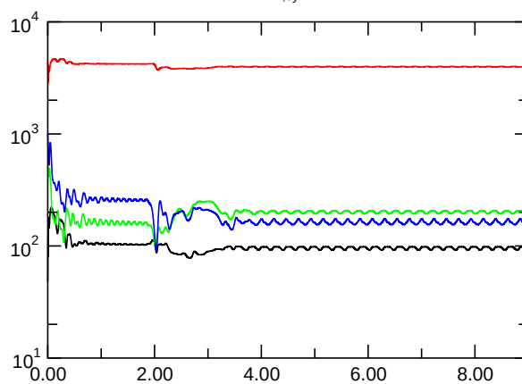
Nusselt Number
