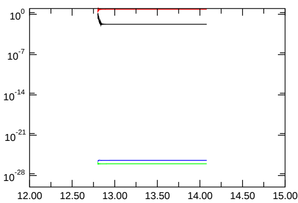
E_{kin,symm.}
