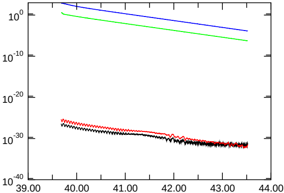
E_{\text{kin,asymm.}}
