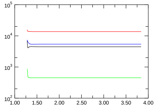
E_{\text{kin,symm.}}
