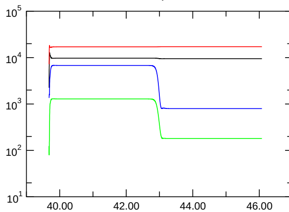
E_{\text{kin,symm.}}
