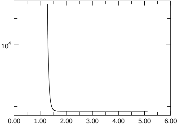
E_{\text{kin,asymm.}}
