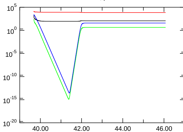
E_{\text{kin,symm.}}
