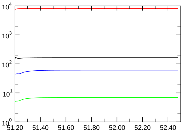
E_{\text{kin,symm.}}
